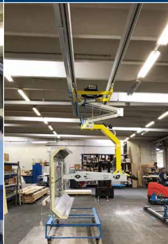
Turning device with load guide Wendegerät mit Lastführung
