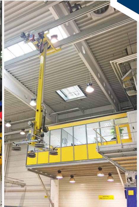
MANIPULATOR FÜR TRIEBWERKS- VERKLEIDUNG
